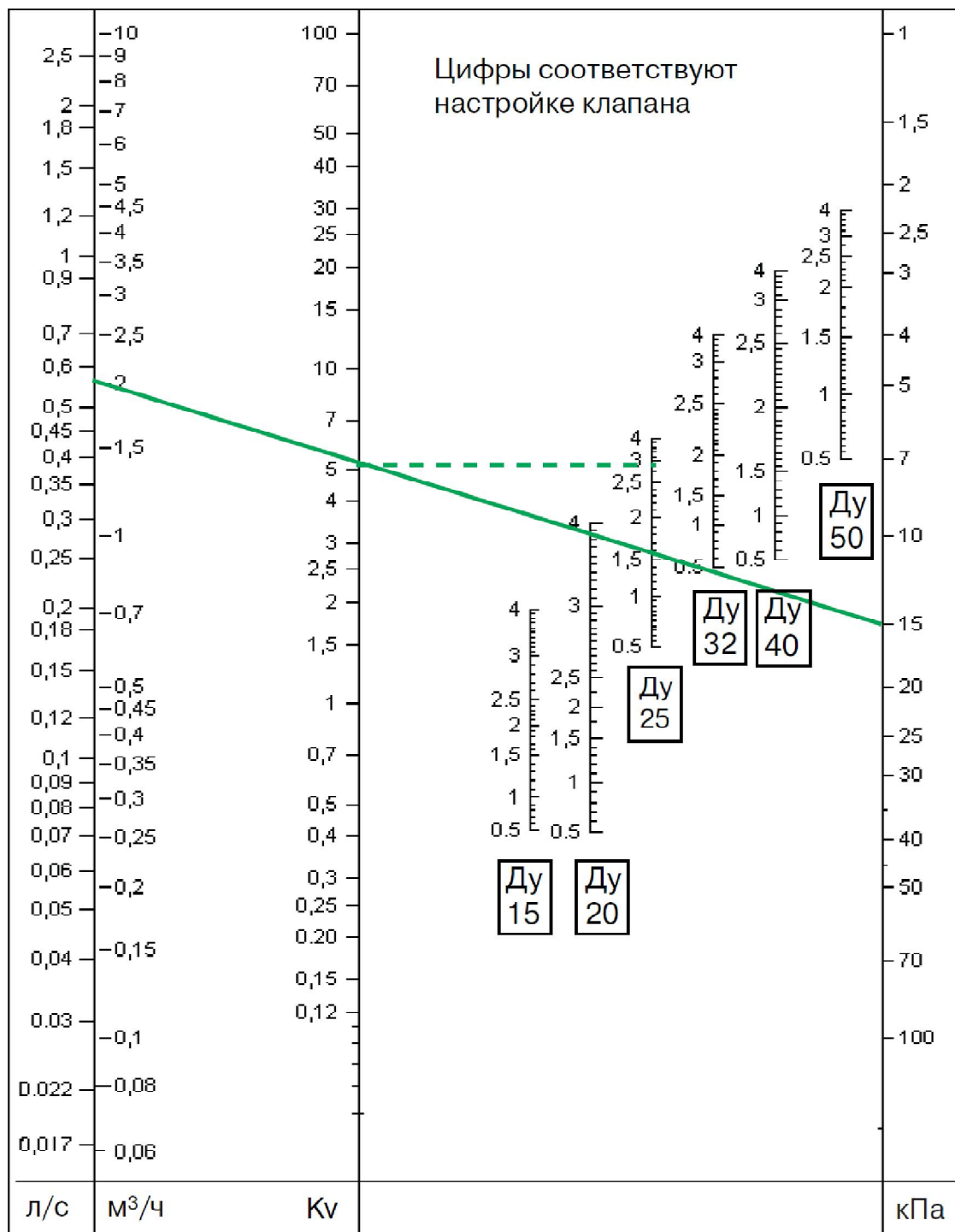
Диаграмма 2. Подбор типоразмера и предварительной настройки клапана
