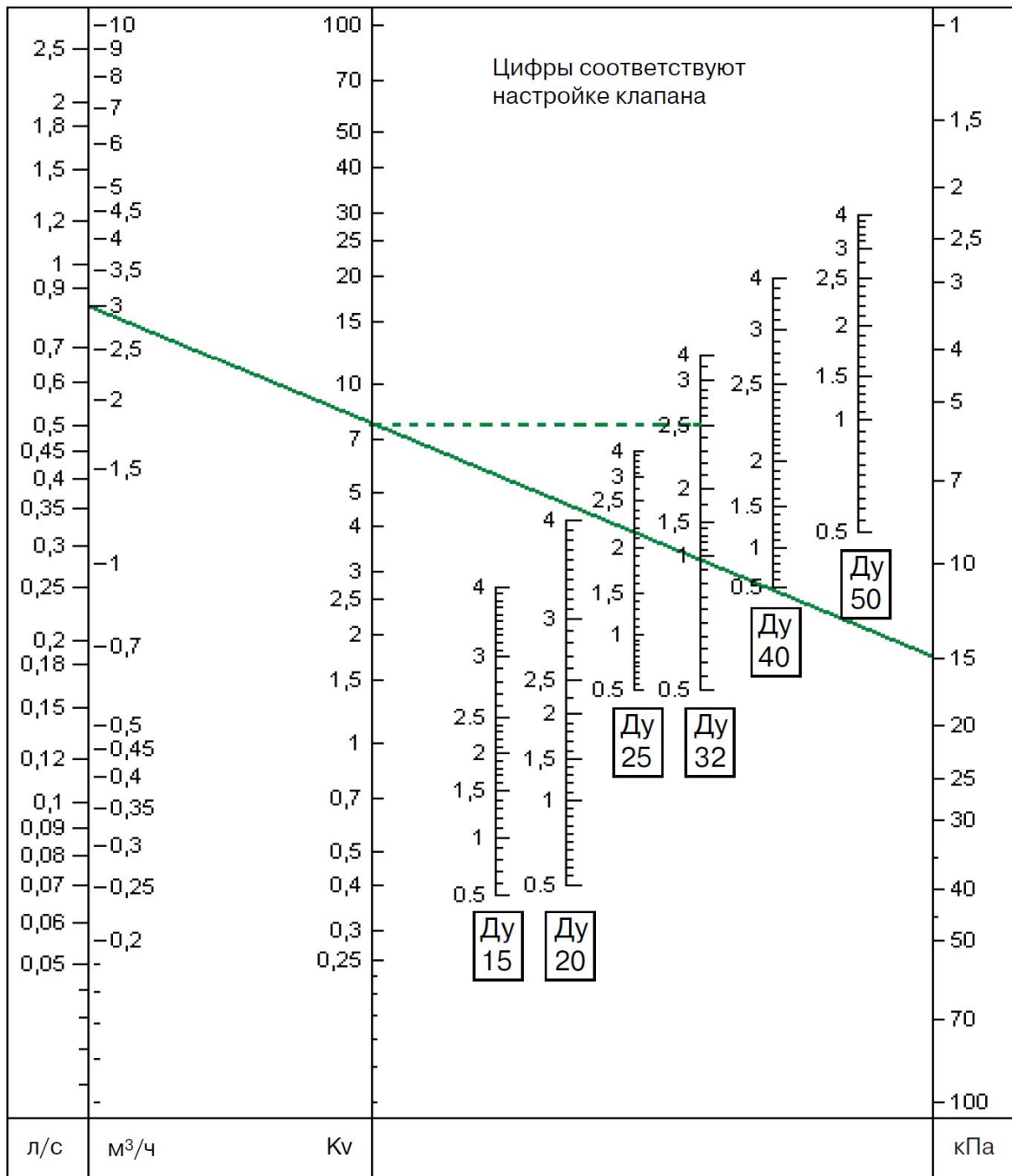
Диаграмма 1. Подбор типоразмера и предварительной настройки клапана
