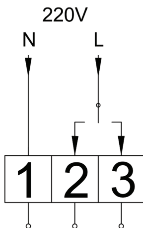
Схема подключения ЭПР-0,6кН
